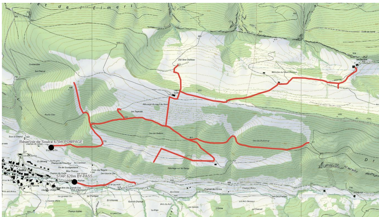
Tracé schématique des nouvelles conduites
