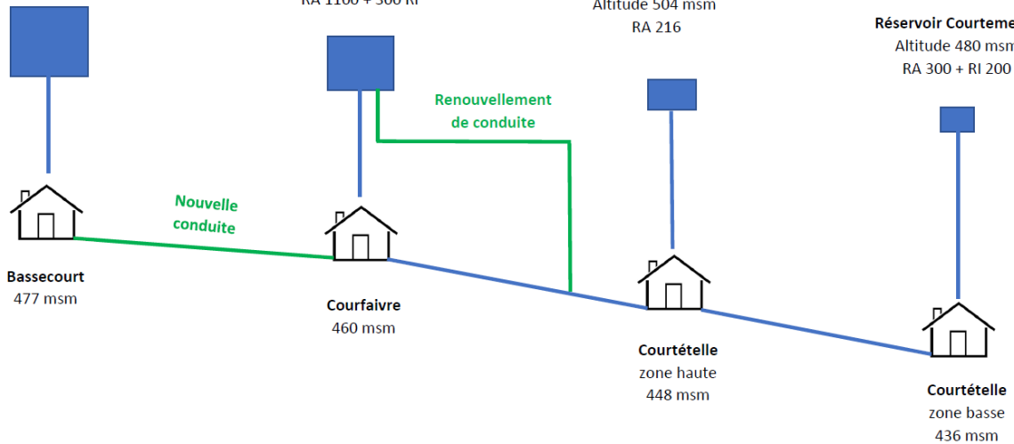
Figure 1 : Vue schématique du réseau hydraulique après travaux
